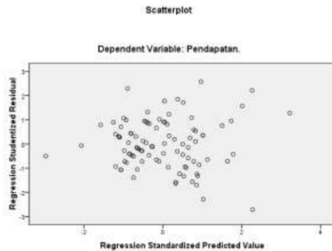
Gambar 2 Uji Heteroskedastisitas
